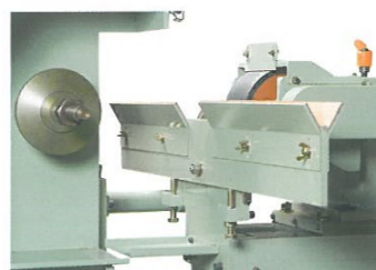
ワーク受台 高さ調整場所 Work rest,height adjusting place.
