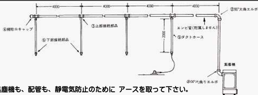
〔配管参考例〕
